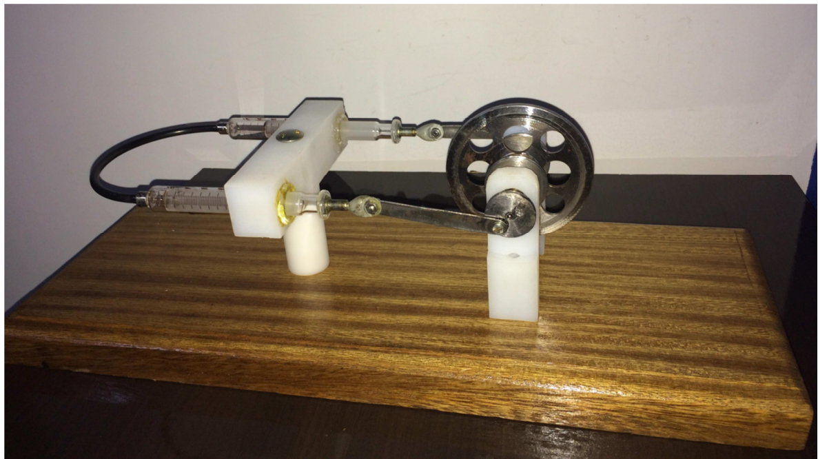
Figura 18 – Motor Stirling modelo Alfa artesanal após a montagem.
